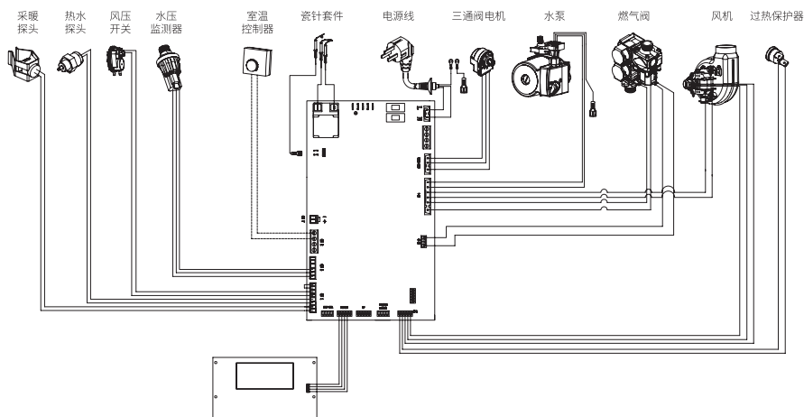
电气接线图
