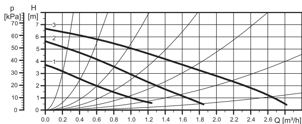
7 米定频水泵特性曲线图
