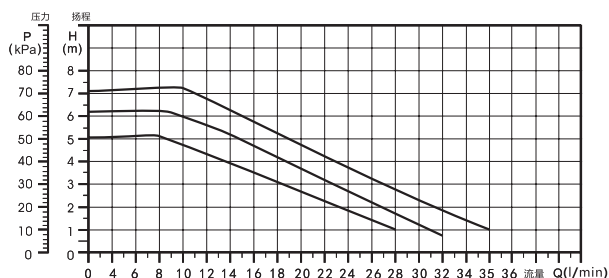
5、6、7 米变频水泵特性曲线图
