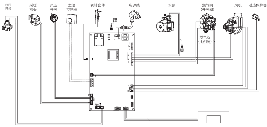
电气接线图
