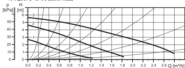
7 米定频水泵特性曲线图
