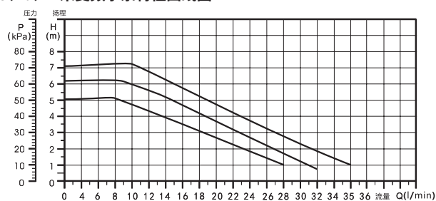
5、6、7 米变频水泵特性曲线图
