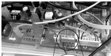
外接室温 控制器
