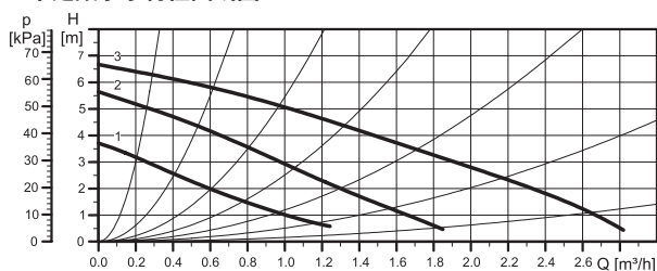
5、6、7 米变频水泵特性曲线图
