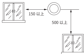
给排气管出口距进风口距离
