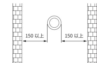
给排气管出口正面
