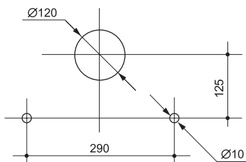
宝石款钻孔尺寸
