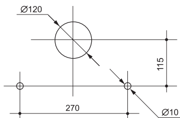
迷你款钻孔尺寸
