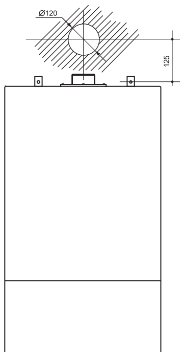
宝石款钻孔尺寸
